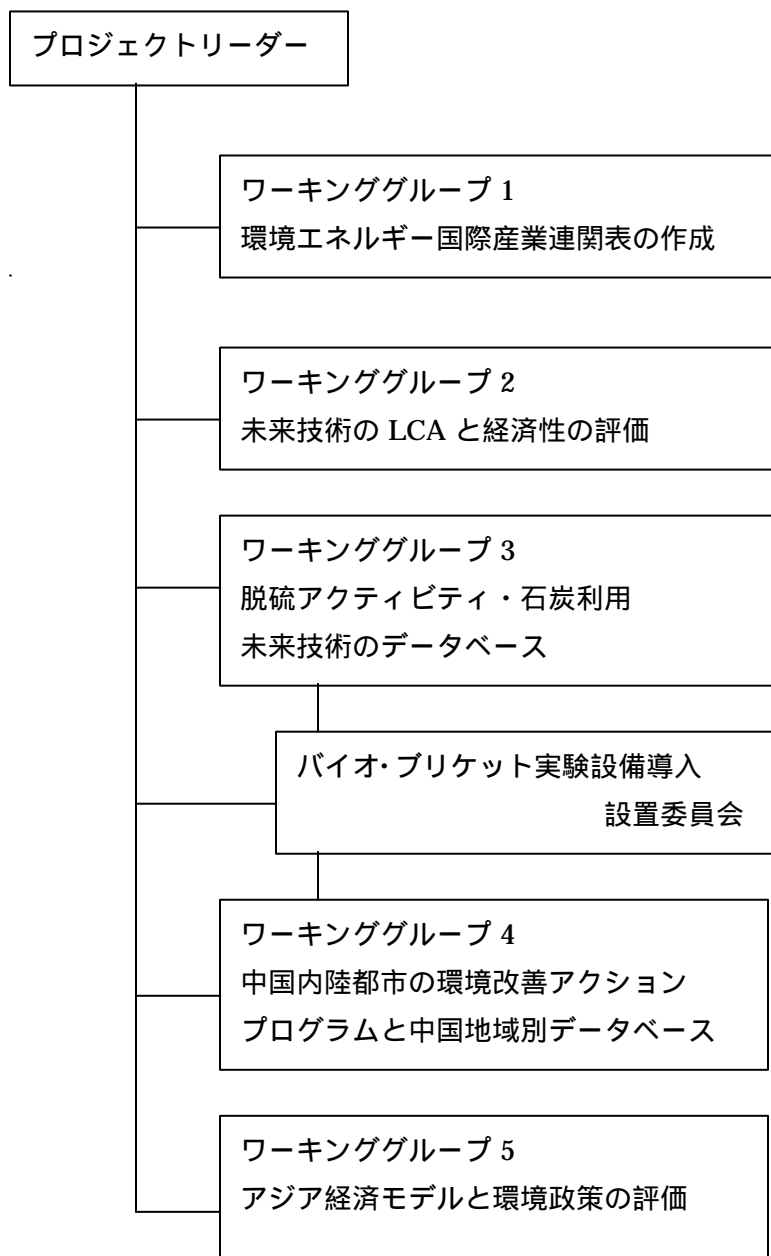
図 3 研究組織図
